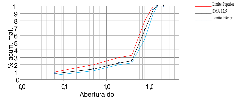
Figura 2: Curva granulométrica da mistura SMA 12,5.
